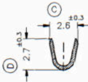
Secc. Z-Z'
