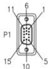
HDB15 M
