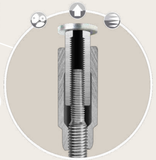
Sistema de embolo con doble rosca.
