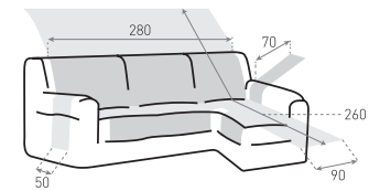
Brazo largo izquierda 280 Long left arm
