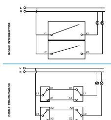
Doble Conmutador / Interruptor
