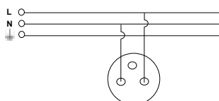
Bases de enchufe
