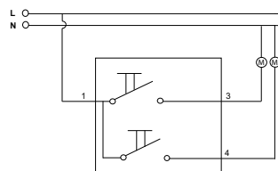
Pulsador de persiana
