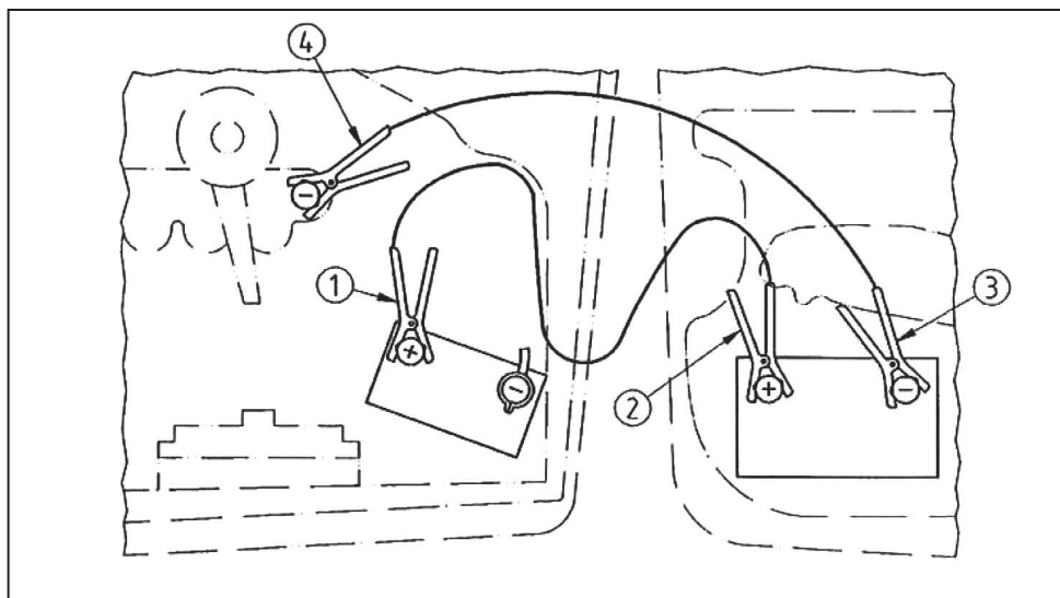
Skeem A.1: Terminaliklambrite ühendamise järjekord
