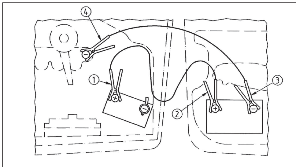
Diagram A.1: Kolejność podłączania zacisków
