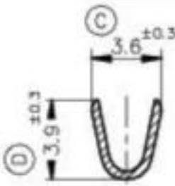
Secc. X-X'
