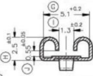
Secc. Z-Z'
