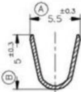
Secc. X-X'
